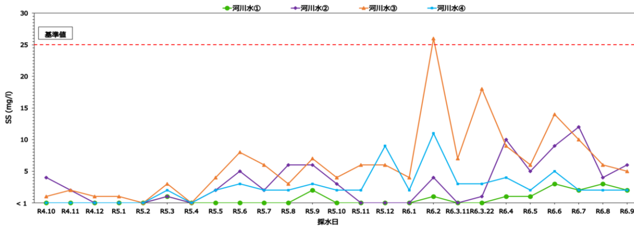
図1: 河川水の測定結果 (SS:浮遊物質量)
